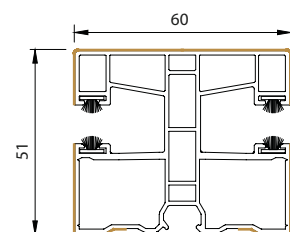
zweiseitige Führungsschiene
