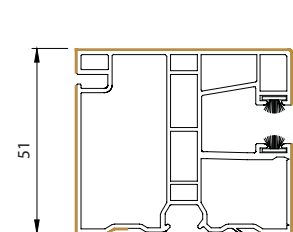
einseitige Führungsschiene
